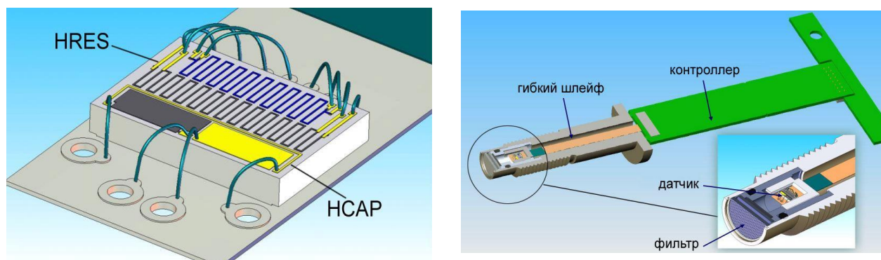
Рис. 2. Схема тонкопленочного датчика MOD- 2740 (HCAP и HRES - емкостная и резистивная часть соответственно) и измерительной ячейки на его основе.
